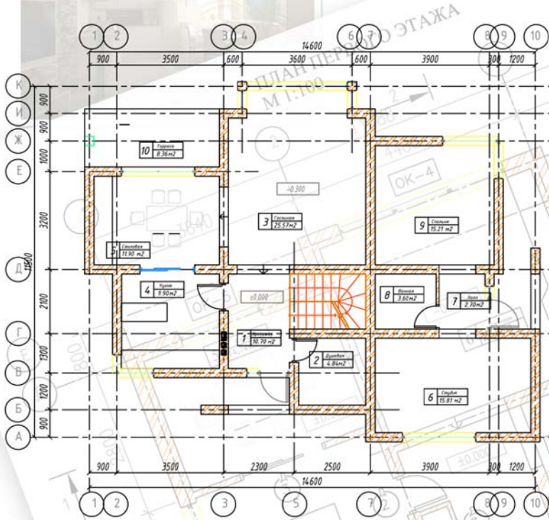
План 1 этажа S=99.32м 2
